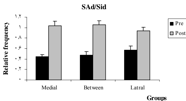
نمودار ۳- مقایسه دوز نقاط جفت نشده، قبل و بعد از اعمال نیم‌بلوک (در روش SAD). دوز نقاط جفت نشده، در هر دو حالت قبل و بعد از اعمال نیم بلوک به دوز نقاط مجاورشان در میدانهای مماسی نرمال گردیده‌اند. Pre: اندازه‌گیری قبل از بکارگیری نیم بلوک Post: اندازه‌گیری بعد از بکارگیری نیم بلوک Medial: نقطه ۱ در شکل (۳-۲b) Lateral: نقطه ۳ در شکل (۳-۲b) Between: نقطه ۲ در شکل (۳-۲b)
