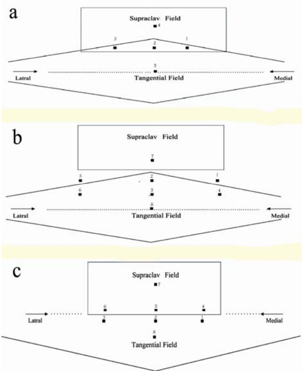
شکل-۱: شمایی از وضعیت میدانهای مماسی و فوق ترقوه نسبت به یکدیگر و موقعیت دزیمترها (a) همپوشانی میدانها در روش SSD (b) جفت شدن میدانها در روش SAD (c) جفت شدن میدانها توسط نیم‌بلوک (Half-block)
