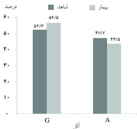
نمودار- ۲: فراوانی آلل‌های پلی‌مورفیسم G/A ۹۷۱- پروموتور ژن CYP2D6 در گروه کنترل و بیمار (P>۰/۰۵).
