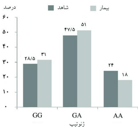
نمودار- ۱: فراوانی ژنوتیپ‌های پلی‌مورفیسم G/A ۹۷۱- پروموتور ژن CYP2D6 در گروه کنترل و بیمار (P>۰/۰۵).
