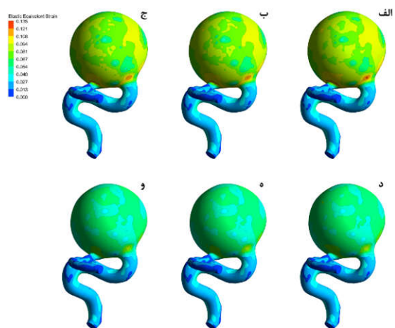
شکل ۵: توزیع کرنش الاستیک در حل جامد نئوهوکین در حل سیال (الف) پاورلا، (ب) کارو، (ج) نیوتنی و حل جامد مونی‌ریولین در حل سیال (د) پاورلا، (ه) کارو و (و) نیوتنی
