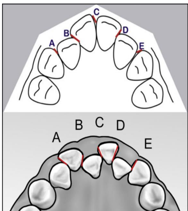
شکل ۲: Little irregularity index در ماگزبلا و مندبیل A+B+C+D+E
