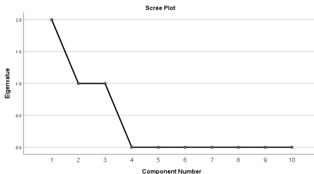
نمودار ۱: نمودار سنگریزه و تعیین نقطه شکست
