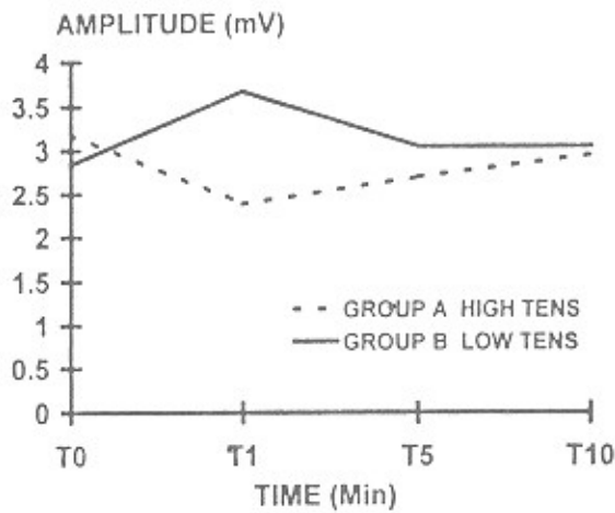
شکل شماره (۱). مقایسه آمپلی تود رفلکس H در زمان های مختلف T0, T1, T5 & T10 در گروه الف HIGH TENS و گروه ب LOW
