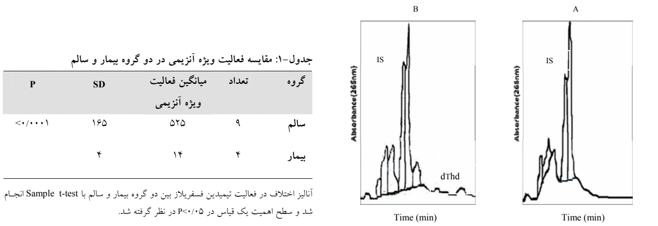
شکل ۲- A: کروماتوگرام فرد سالم: پیک تیمیدین دیده نمی‌شود. B: کروماتوگرام فرد بیمار: دارای پیک تیمیدین در پلاسما
