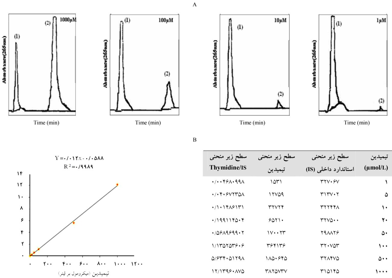
شکل ۱- A: کروماتوگرام‌های تیمیدین نمونه‌های استاندارد در غلظت‌های ۱، ۵، ۱۰، ۲۰، ۵۰، ۱۰۰، ۵۰۰ و ۱۰۰۰ میکرومولار. کروماتوگرام‌های ۱، ۱۰، ۱۰۰ و ۱۰۰۰ (۱: پیک استاندارد داخلی ۲: پیک استاندارد خارجی). B: منحنی استاندارد تیمیدین مورد استفاده برای تبدیل اعداد مربوط به سطح زیر منحنی در نمونه‌های مجهول به غلظت‌های میکرومولار تیمیدین
