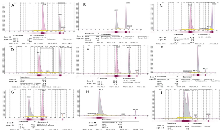
شکل ۲: الکتروفورگرام مربوط به واریانت‌های زنجیره بتا. مطابق الکتروفورگرام‌های A و B هموگلوبین E به‌طور کامل در حالت هتروزیگوت و هموزیگوت جدا شده و دارای علامه هماتولوژیکی می‌باشند. اشکال C و D حالت هتروزیگوت هموگلوبین‌های C و O را نشان می‌دهند که با هموگلوبین A 2 تداخل دارند. هموگلوبین D با روش کاپیلاری الکتروفورز به راحتی جدا می‌شود (E و F) هموگلوبین J در صورت همراهی با بتا تالاسمی هتروزیگوت (مینور)، بیشترین درصد هموگلوبین را تشکیل می‌دهد (G, H). هموگلوبین Hope کمی سریع‌تر از هموگلوبین A حرکت کرده و در ناحیه ۱۰ الکتروفورگرام قرار می‌گیرد (J).
