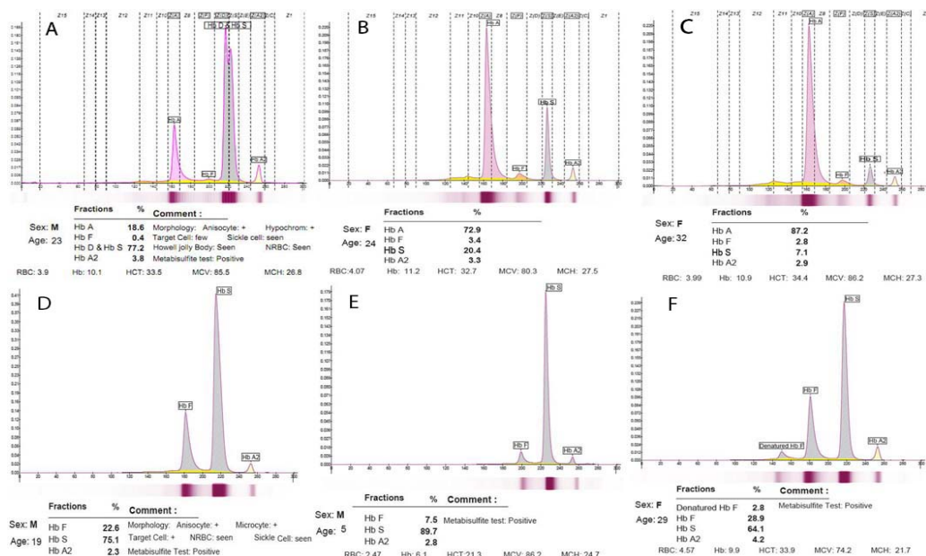
شکل ۳: الکتروفورگرام‌های مربوط به اشکال مختلف هموگلوبین S با روش کاپیلاری الکتروفورز. در حالت ترکیبی S و D، دو هموگلوبین از هم جدا نمی‌شوند (A). به‌طور معمول در حالت هتروزیگوت حدود ۴۰٪ هموگلوبین S وجود دارد در حالی که براساس الکتروفورگرام‌های B و C درصد پای‌تری ممکن است مشاهده شود که بایستی با تست‌های مولکولی تایید شود. در حالت هموزیگوت هموگلوبین S و یا همراهی با تالاسمی مینور، پیک هموگلوبین A وجود ندارد (D, E, F).
