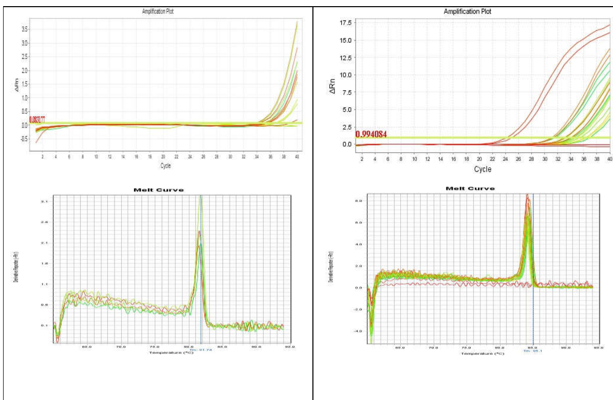
شکل ۱: سیکل دمایی و منحنی ذوب برای ژن بتا اکتین (سمت راست) و آلکالین فسفاتاز (سمت چپ) لنفوسیتی.
