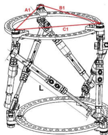
شکل ۲: نحوه اندازه‌گیری‌ها
