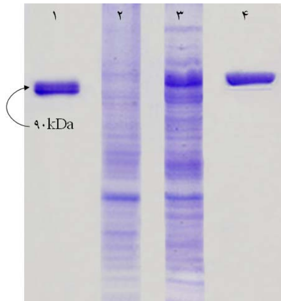
شکل ۲: الگوی الکتروفورزی نمونه‌های پروتئینی در طول خالص‌سازی ۱: مارکر وزن ملکولی ۲: باکتری BL21 بدون پلاسמיד ۳: عصاره خام باکتری قبل از خالص‌سازی ۴: SK-MBP خالص شده
