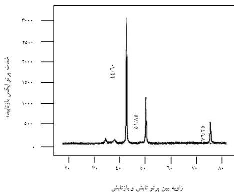
نمودار ۱: نمودار پراش پرتوی ایکس از نانوذرات ۴۰ و ۸۰ nm طیف XRD نانوذرات به‌دست آمده در زوایای ۵۱/۸۵، ۷۶/۲۵ و ۷۶/۲ مربوط به پراش از صفحات بلوری نانوذرات مس می‌باشد.
