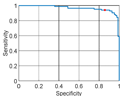
شکل ۲: منحنی ROC عملکرد مدل پیشنهادی بر روی داده‌های تست. نقطه قرمز نشانگر نتایج با آستانه اطمینان طبقه‌بندی 0.5 است.
