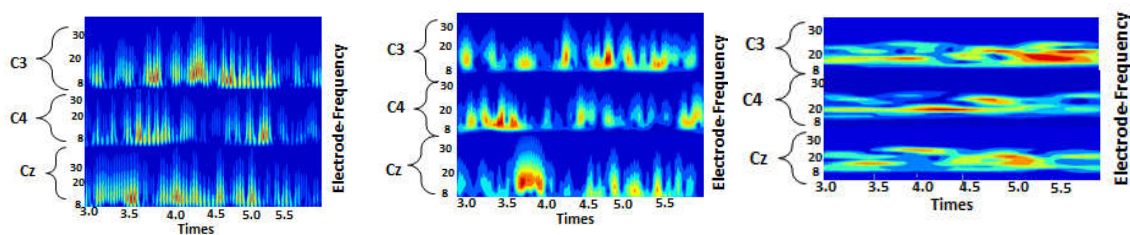
شکل ۳: نمونه تبدیل موجک یک داده زمانی در سه کانال منتخب C3، C4 و Cz با موجک‌های مادر مختلف، از سمت چپ به ترتیب Cmor، Mexicanhat و Cgaus
