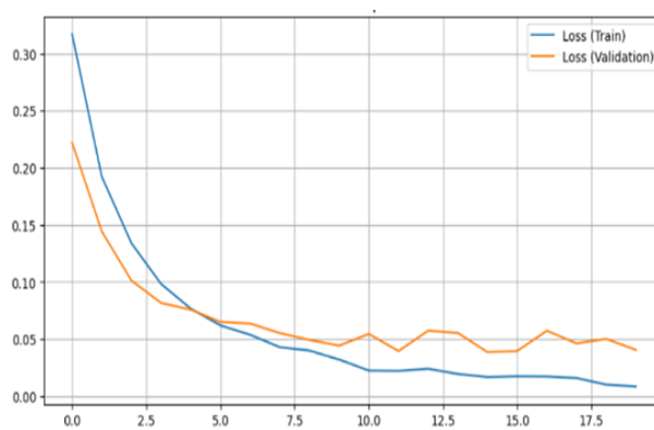
شکل ۵: نمودار خطا (زیان) بر حسب اپاک.
