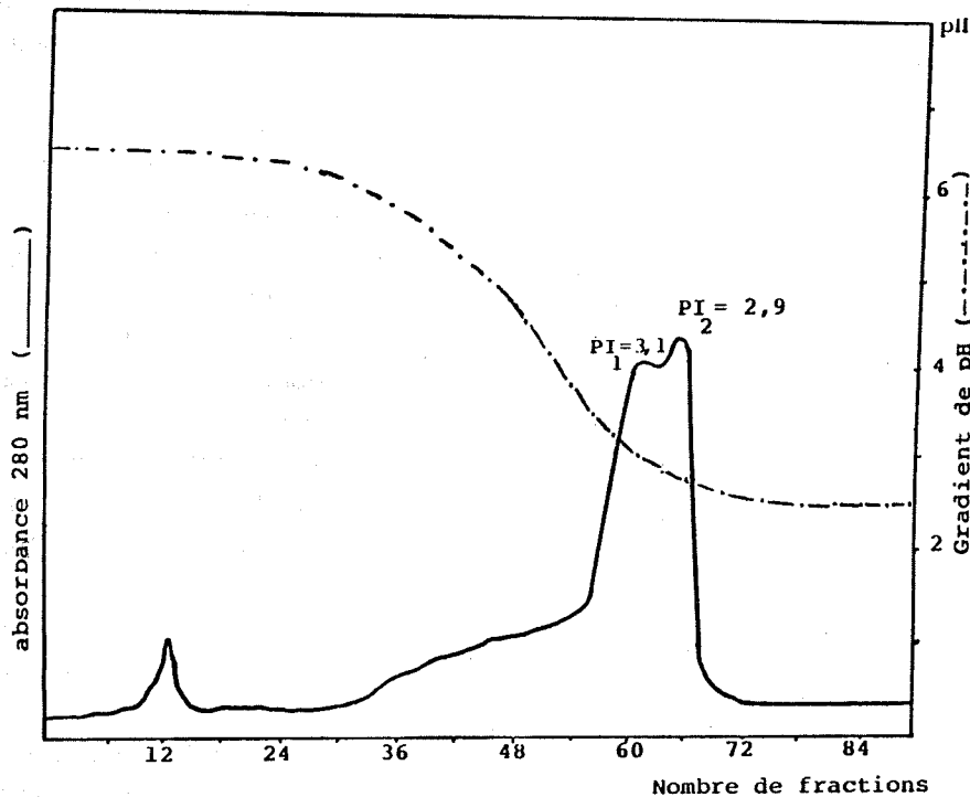
نمودار ۳- کروماتوگراف کالیزاسیون تعویض یونی با گرادیان pH ۶/۳ تا ۲/۵
