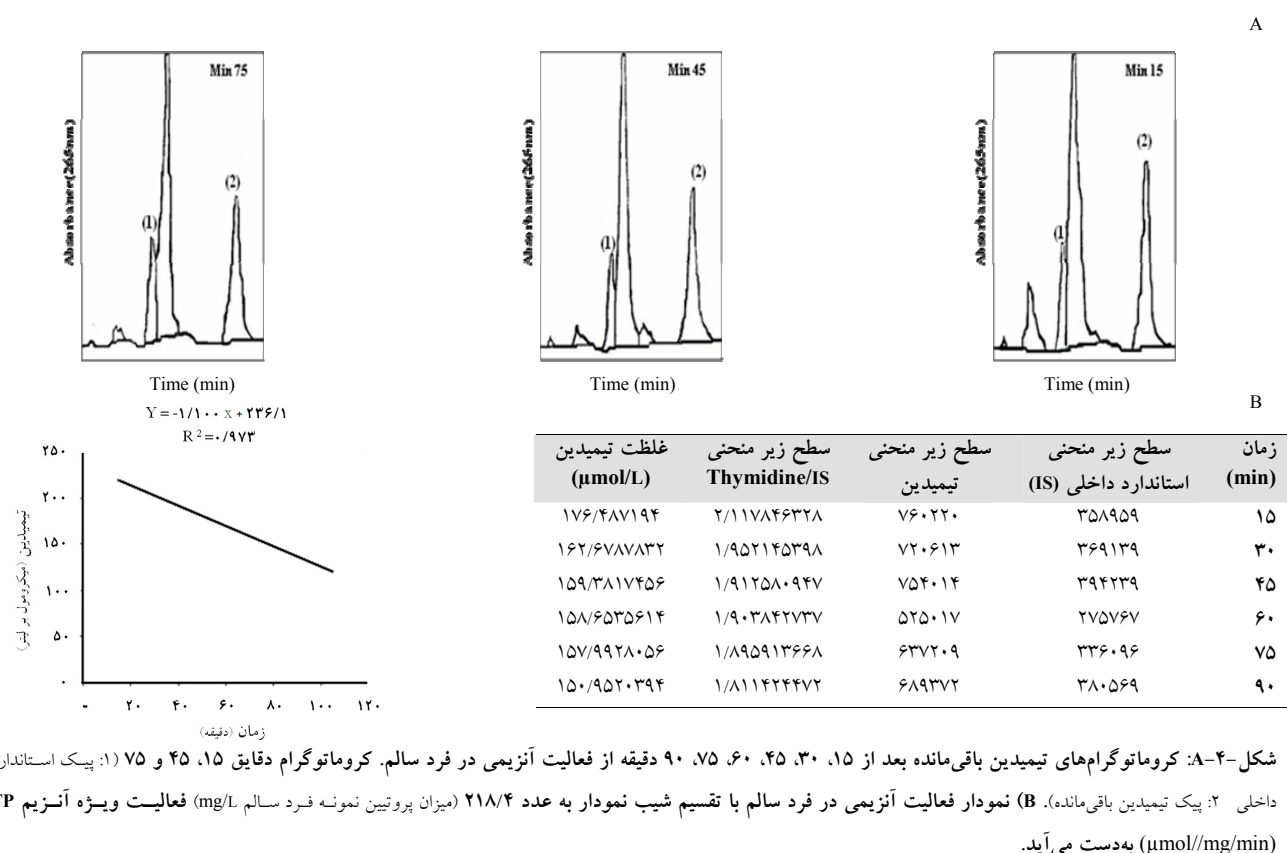
شکل ۳- A: کروماتوگرام‌های تیمیدین باقی‌مانده بعد از ۱۵، ۳۰، ۴۵، ۶۰، ۷۵، ۹۰ دقیقه از فعالیت آنزیم در یک بیمار. کروماتوگرام دقایق ۱۵، ۴۵ و ۷۵: ۱) پیک استاندارد داخلی ۲: پیک تیمیدین باقی‌مانده. (B) نمودار فعالیت آنزیمی در بیمار با تقسیم شیب نمودار به عدد ۲۸۲/۸ (میزان پروتیین نمونه بیمار mg/L) فعالیت ویژه آنزیمی (μmol/mg/min) به‌دست می‌آید.
