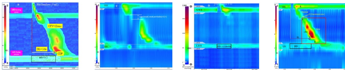
شکل ۲: (A) نمونه‌ای از توپوگرافی فشار مری، (B) عدم کامل انقباض، (C) انقباض ضعیف با بریدگی بزرگ، (D) اسپاسم دیستال مری با DL کمتر از ۴/۵ ثانیه A: زمان در محور افقی و فاصله از سوخاخ بینی در محور عمودی نمایش داده شده است. دو ناحیه پر فشار در تصویر دیده می‌شود که در بالا اسفنکتر فوقانی (UES) و در پایین اسفنکتر تحتانی (LES) است. فشار شل شدن کامل اسفنکتر فوقانی و تحتانی در چهار ثانیه (IRP4) با تعیین میانگین پایین‌ترین فشار شل شدن اسفنکتر در چهار ثانیه محاسبه می‌گردد. ناحیه‌ای از لوله مری است که از آمپول فرنیک جدا می‌شود و فشار ۳۰ mmHg به‌طور ناگهان تغییر می‌کند. Contractile front velocity (CFV)، سرعت (Velocity) نیروی انقباضی که از طریق مناسب‌ترین تانژانت زاویه بین نقاط P و Contractile deceleration point (CDP) طرح هم‌فشار (ایزو باریک) ۳۰ mmHg محاسبه می‌شود. Distal latency (DL) تاخیر انقباض بخش دیستال مری، با فاصله بین شل شدن اسفنکتر فوقانی و CDP و بر حسب cm تعیین می‌شود و به حاصل ضرب آهلی تود، مدت و طول انقباض بخش دیستال مری از نقطه P تا D با فشار بیشتر ۲۰ mmHg محاسبه و بر حسب میلی‌متر جیوه‌ثانیه‌سانی متر نمایش داده می‌شود و به‌نام انقباض کامل دیستال مری (Contractile deceleration point, DCI) نامیده می‌شود.
