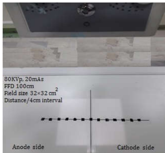
شکل ۱: اندازه‌گیری پروفایل تغییرات شدت اشعه به صورت تجربی بدون حضور بیمار (در هوا) در راستای محور مرکزی بین کاتد-آند در فاصله ۱۰۰ cm از تیوب.
